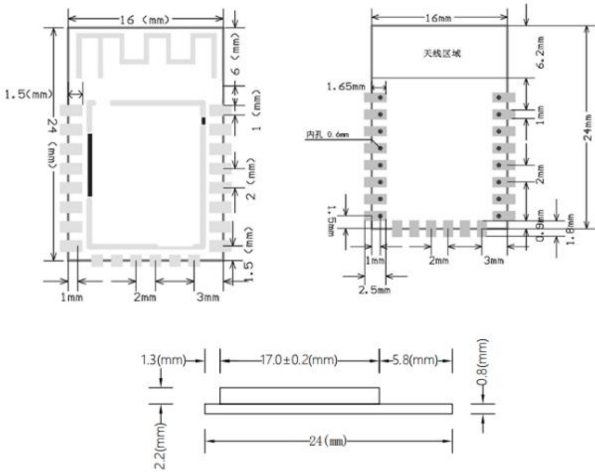
图4: WG236 参考 PCB 封装/Recommend PCB Footprint
