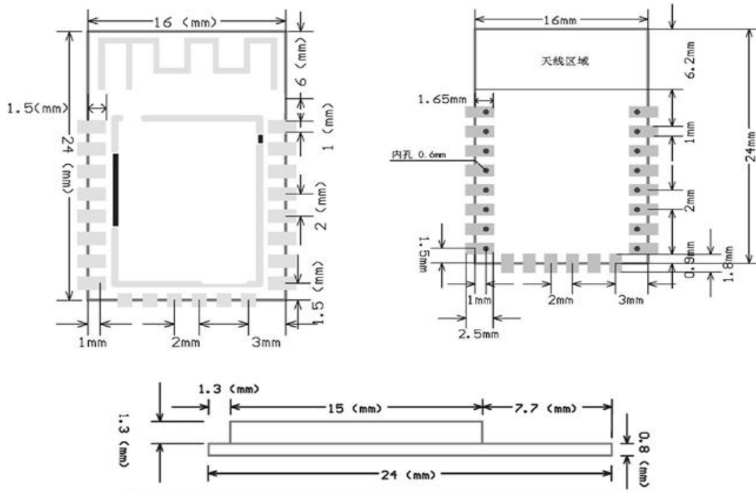
图4: WG236 参考 PCB 封装/Recommend PCB Footprint
