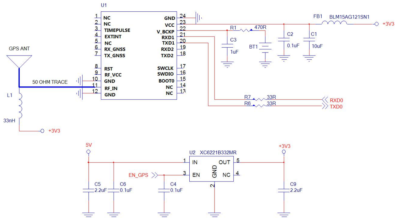
图 5: SKM-4DU 参考电路
