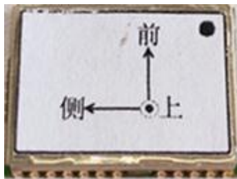
图 7: SKM-4DU 安装方式
