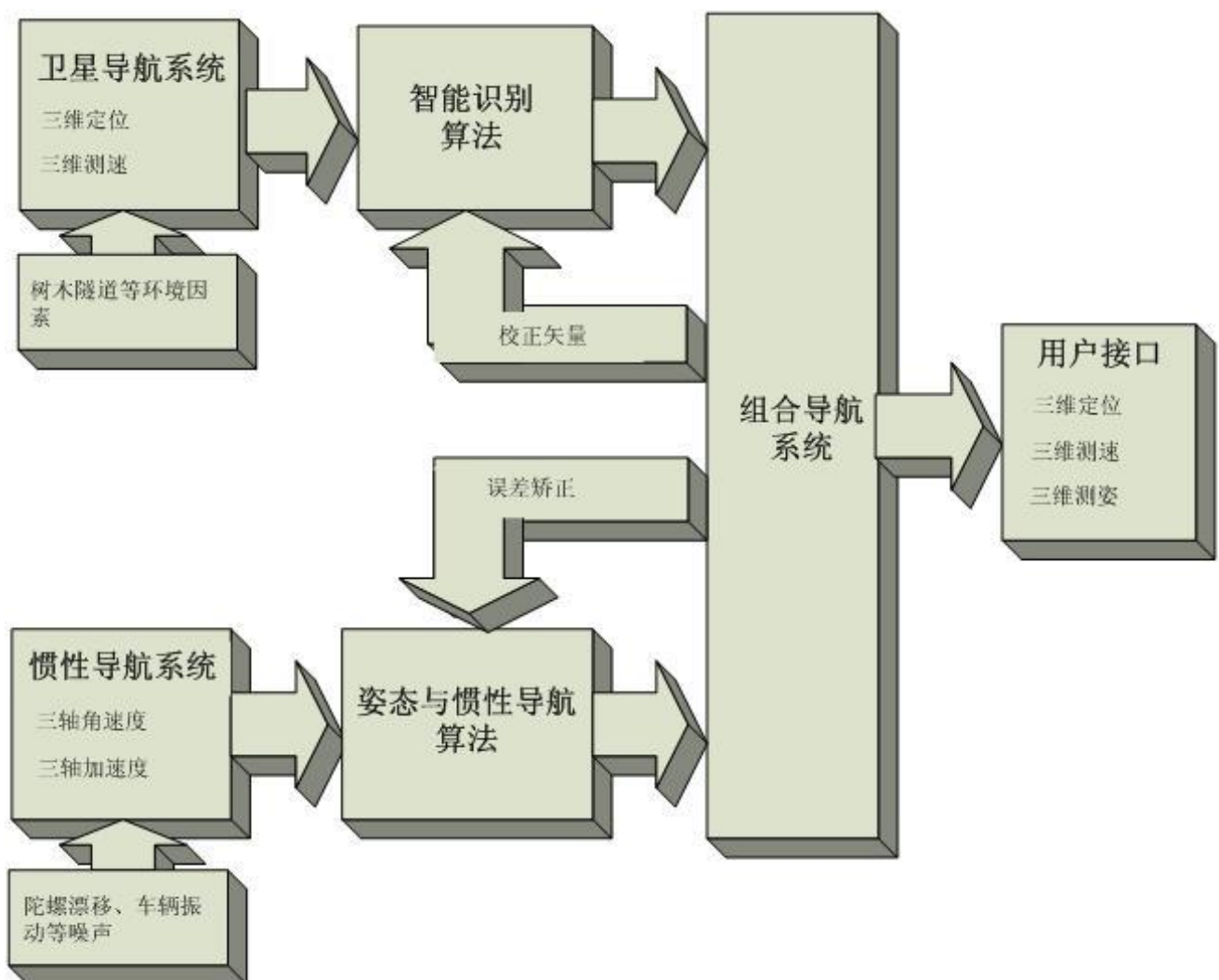
图 2: SKM-4DU 设计原理图
