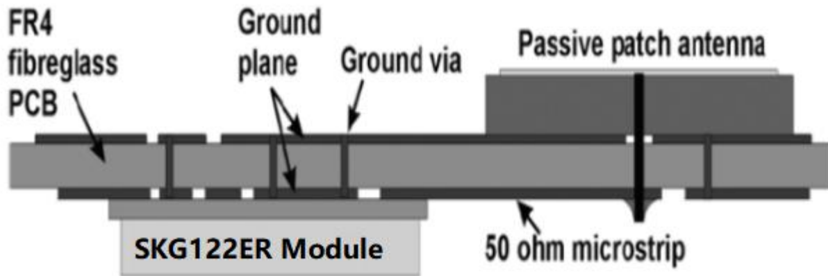
图 11.1-1 SKG122ER 参考设计/ Figure 11.1-1 SKG122ER reference design
