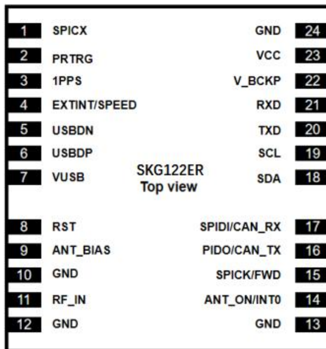
图 5-1 SKG122ER 引脚定义/ Figure 5-1 SKG122ER pin definitions
